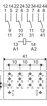
56.44 Ansicht auf die Anschlüsse
