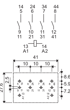
56.44-0300 Ansicht auf die Anschlüsse
