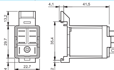
056.27 mit Relais
