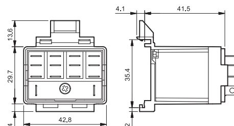
056.47 mit Relais
