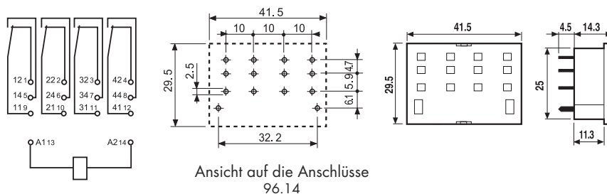
Ansicht auf die Anschlüsse 96.12
