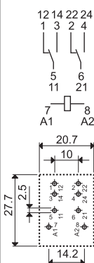
56.42 Ansicht auf die Anschlüsse
