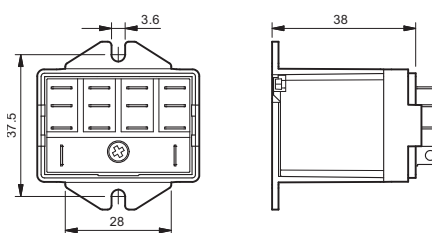
056.45 mit Relais
