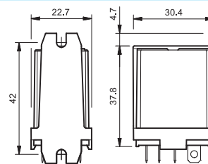
056.26 mit Relais
