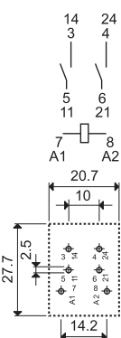
56.42-0300 Ansicht auf die Anschlüsse
