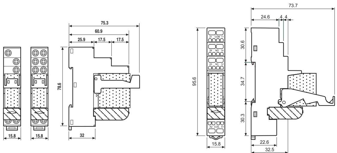
48.31 48.52 / 48.61 / 48.62 Schraubklemmen
