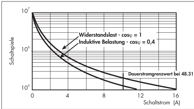
F 48 - Elektrische Lebensdauer bei AC Typ 48.31/61/81
